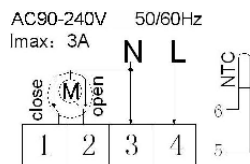
Veden lämmityksen kytkentäkaavio (älä kytke sähköventtiiliin liitintä "close 4")
