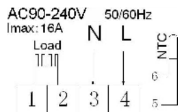
Sähkölämmityksen kytkentäkaavio
