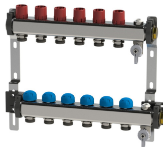
Lattialämmitysjakotukki - yksi toimilaite per sinisen käsisäätöpyöän tilalle
